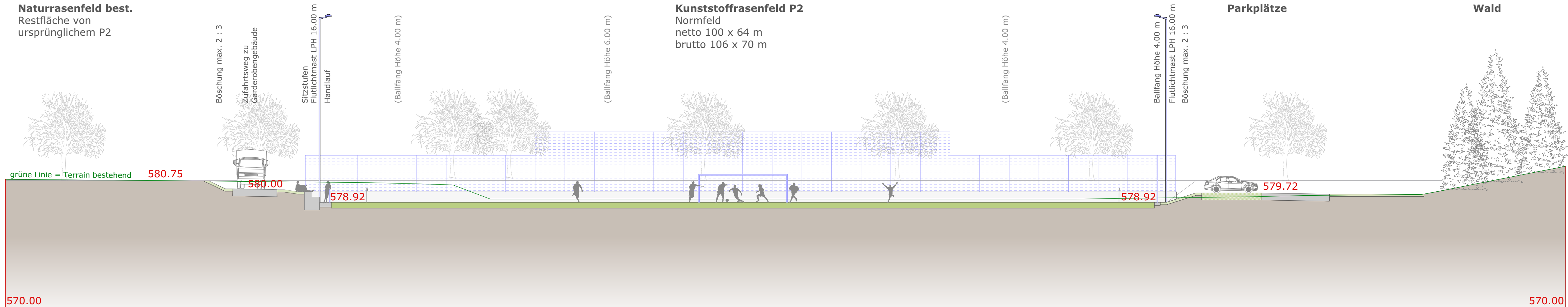
SCHNITT D - D'
