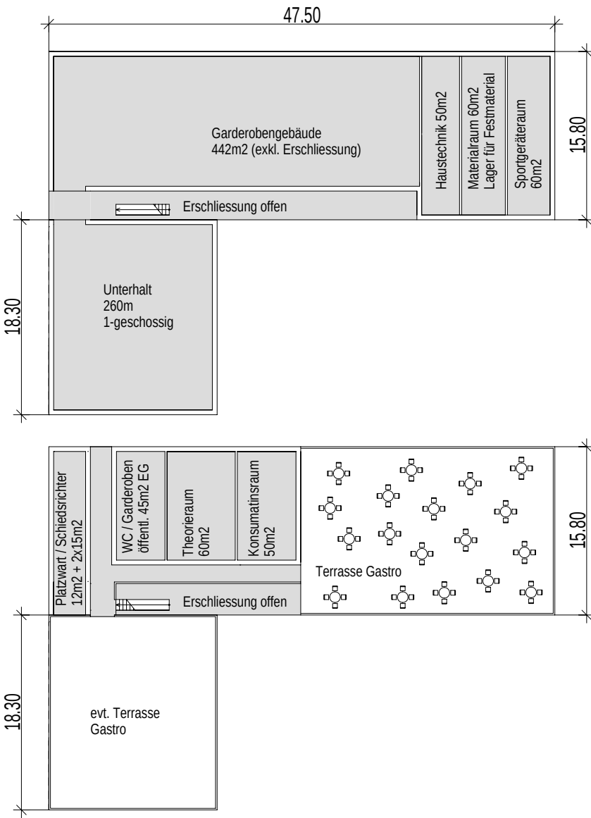
Gartenobergebäude und Unterhaltsgebäude Anordnung Var. E
